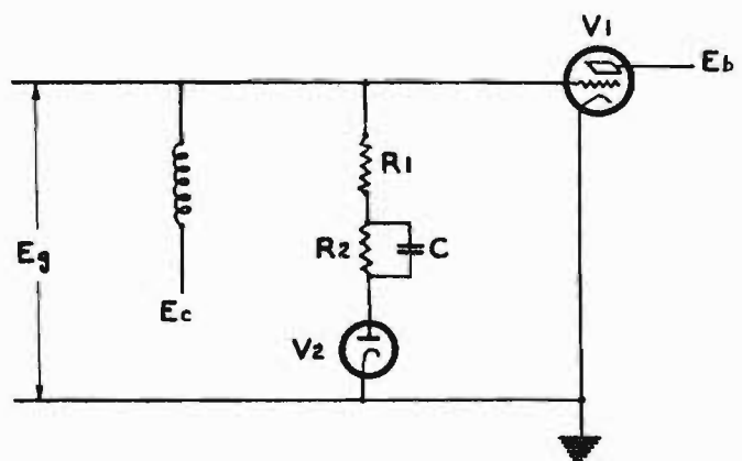
Fig. 3 Dynatron Rectifier
